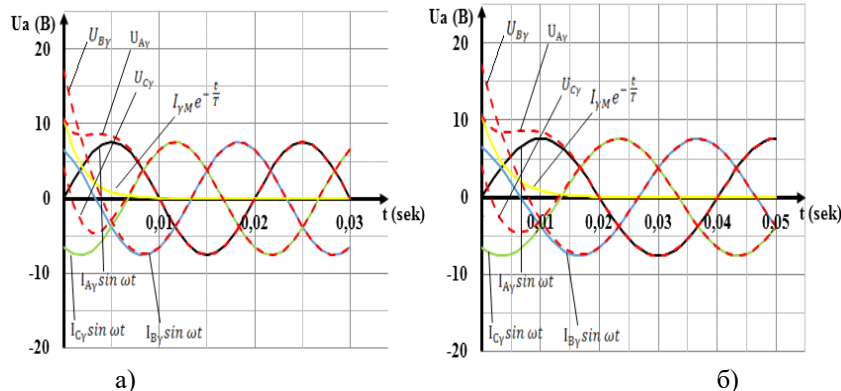
1-расм. Датчикнинг кўп фазали тоқлар ва чиқиш кучланиши орасидаги боғлиқликнинг динамик тавсифлари. (реактив қувват манбалари юлдузсимон уланганда) t=0,02 сония бўлганда холда б) t=0,04 сония бўлганда холда).
