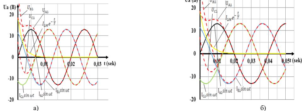
2-расм. Датчикнинг кўп фазали тоқлар ва чиқиш кучланиши орасидаги боғлиқликнинг динамик тавсифлари. (реактив қувват манбалари учбурчаксимон уланганда) t=0,02 сония бўлганда холда б) t=0,04 сония бўлганда холда).
