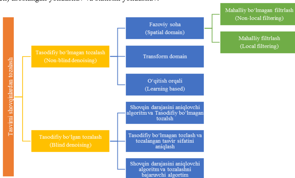
5-rasm. Tasvirlarni shovqinlardan tozalash usullari.
