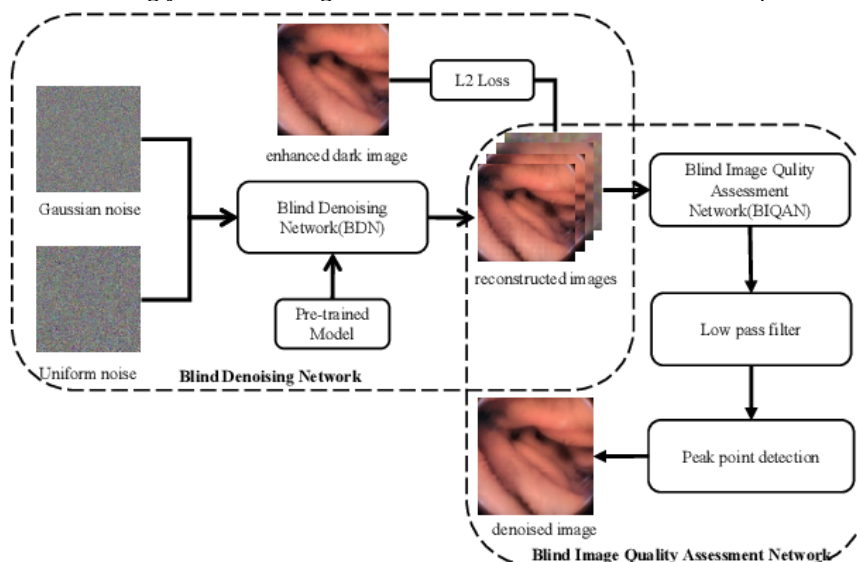
6-rasm. BDN va BIQAN arxitekturalari.
