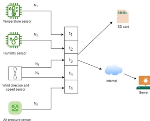
Расм 2. Сенсорлардан олинган маълумотларни вақт бўйича бирлаштириш усули.
