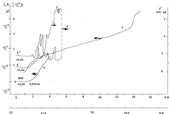
6-Расм. Кремнийли р-п ўтишда ВАХ нинг модуляциявий дифференциаллаш методи ёрдамида олинган типик боғланишлар [15].
