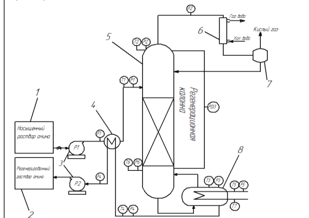
Рис.2. Принципиальная схема экспериментальной лабораторной установки для регенерации амина.
