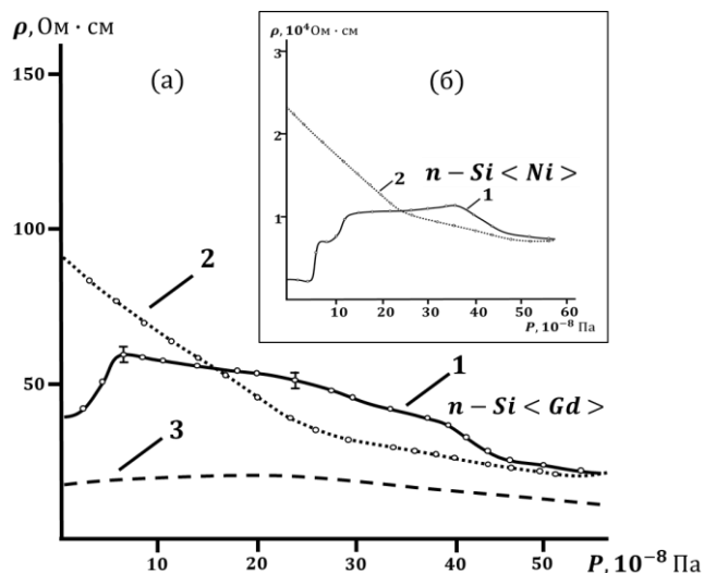
Рис. 2 Тензосопротивление образцов (а) – n\text{-Si}<\text{Gd}> и (б) – n\text{-Si}<\text{Ni}> при всестороннем гидростатическом сжатии (1 – с увеличением P , 2 – с уменьшением P , 3 – n\text{-Si} )
