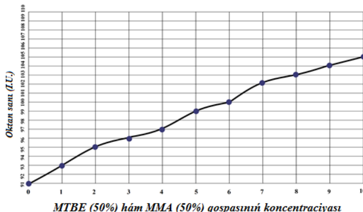
3-súwret. MTBE (50%) hám MMA (50%) qospasınıń jergilikli AI-91 benziniń oktan sanın asırıw dárejesi
