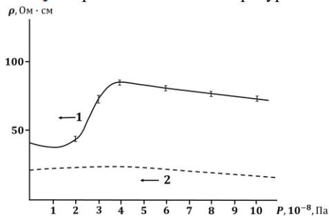
Рис. 1 Зависимость \rho от P для образцов n\text{-Si}<\text{Gd}> (крив. 1) и для n\text{-Si} (крив. 2) при ВГД.
