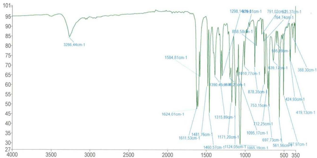
1-rasm. Indigoning IQ-spektri
