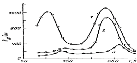
3-Расм. Ҳар хил температураларда кремнийли р-п ўтишдаги дифференциаль қаршилиқнинг температурага боғлиқлиги [2].
