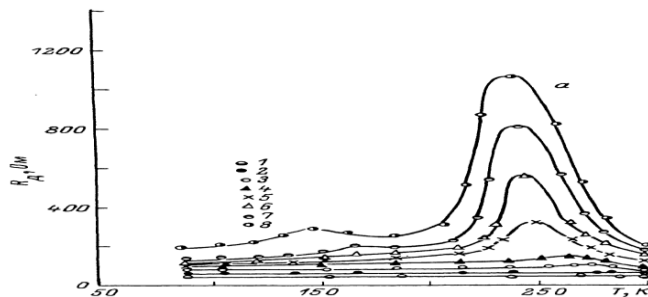
1-Расм. Кремнийли р-п тескари утишида пробой саҳосидаги дифференциаль қаршилигининг температурага боғлиқлиги. Флюенс нурланиши, \Phi , \text{см}^{-2} : 1 — нурланишгача, 2 — 5 \cdot 10^{15} , 3 — 1 \cdot 10^{16} , 4 — 2 \cdot 10^{16} , 5 — 3 \cdot 10^{16} , 6 — 5 \cdot 10^{16} , 7 — 4 \cdot 10^{16} , 8 — 6 \cdot 10^{16} [2].
