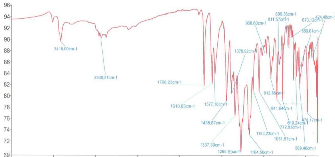
2-rasm. Gossipolsirka kislotasining IQ-spektri
