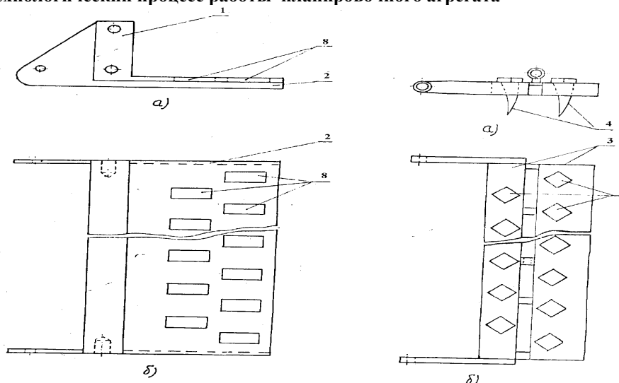
Рисунок 2. Схема рабочего органа и основания мала - планировщика
