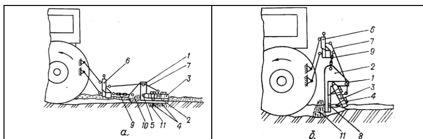
Рисунок 1. Технологический процесс работы планировочного агрегата
