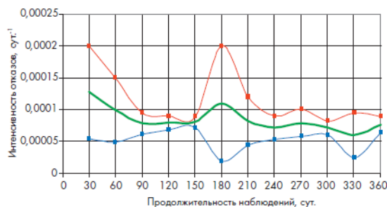
Рисунок 4. Распределение интенсивностей отказов поплавковых клапанов
