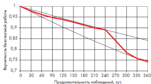
Рис.3. Распределение вероятности безотказной работы смесителей во времени
