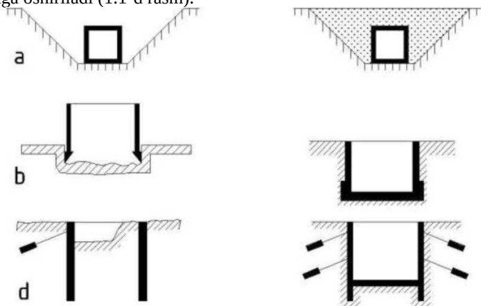
1.1-rasm. Yer osti inshootlarini yer sirtidan barpo etish: a -xandaq usuli; b -pastlashuvchi quduq usuli; d- "grunt qa'rida devor" usuli. I-II - qurilish bosqichlari
