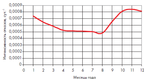
Рис.2. Изменение интенсивности отказов смесителей в эксплуатационных условиях
