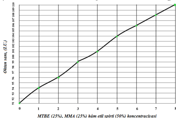
3-súwret. MTBE (25%), MMA (25%) ham etil spirti (50%) qospasınıñ jergilikli AI-91 benzininiñ oktan sanın asırıw dárejesi
