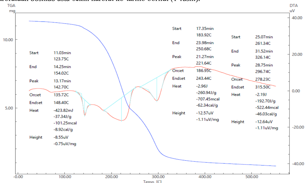
1-rasm. KFA ning termogravimetrik (TGA) va differensial termo analizi (DTA)
