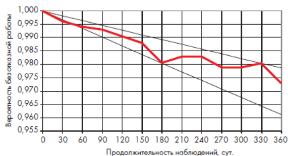
Рисунок 5. Изменение вероятности безотказной работы поплавковых клапанов
