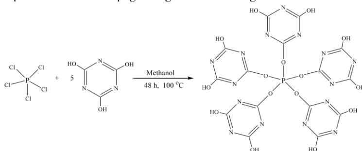
1-sxema. Quramında fosfor saqlaǵan oligomer PSK-1 sintezi.
