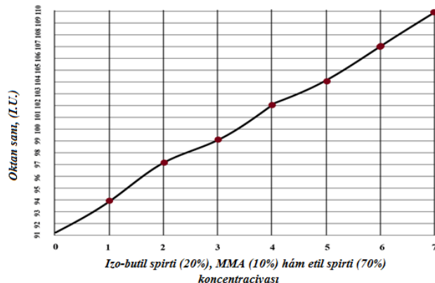
2-súwret. Izo-butil spirti (20%), MMA (10%) ham etil spirti (70%) qospasınıñ jergilikli AI-91 benzininiñ oktan sanın asırıw dárejesi
