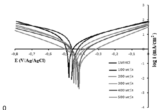
1-súwret. 298 K de PSK-1 diń hár túrli koncentraciyalarda ingibirlengen hám ingibirlenbegen 1M HCl da uglerodli polattıń polyarizaciya iymek sıyıqları.
