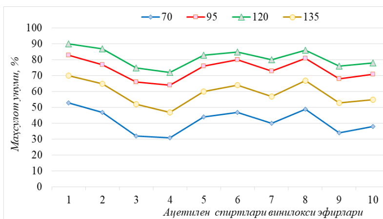
1-Расм. Ацетилен спиртлари винилокси эфирлари унумига ҳарорат таъсири (эритувчи ДМСО, реакция давомийлиги 8 соат, каталитик система- NaOH·CsF, бошланғич маҳсулотлар эквимоляр нисбатда)
