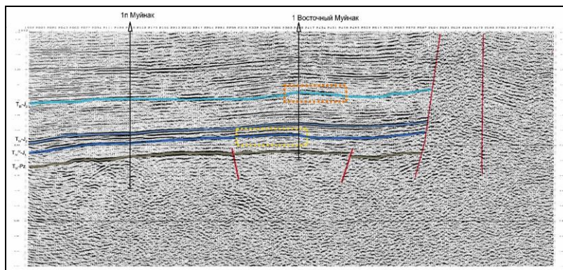
Рис. 1. Фрагмент временного разреза, отражающего строение площади Восточный Муйнак (пунктиром показаны сводовые части ловушки по различным горизонтам юрских отложений)
