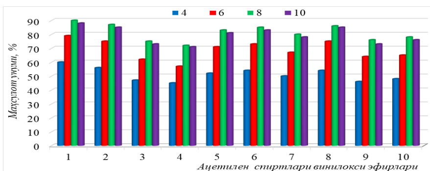
2-Расм. Ацетилен спиртлари винилокси эфирлари унумига реакция давомийлиги таъсири (ҳарорат 120 °С, эритувчи ДМСО, каталитик система- NaOH·CsF)
